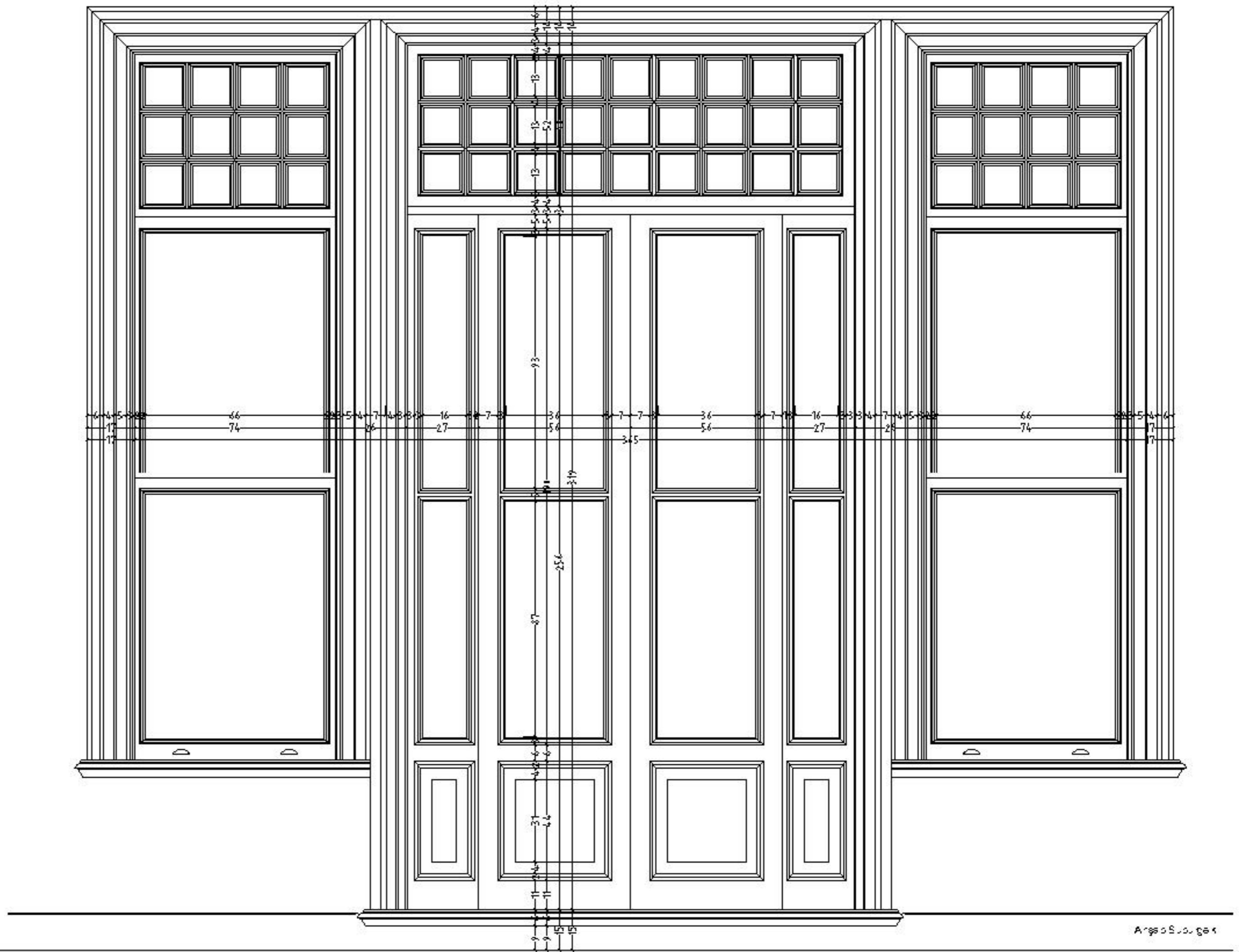
İÇ GÖRÜNÜŞ
