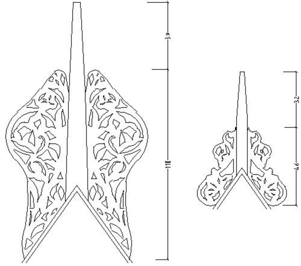
DETAYLAR ÖLÇEK: 1/10
